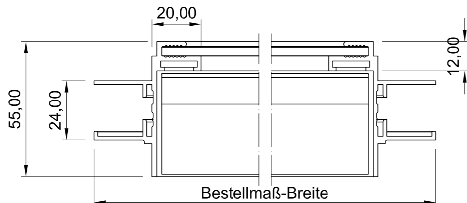
Draufsicht
