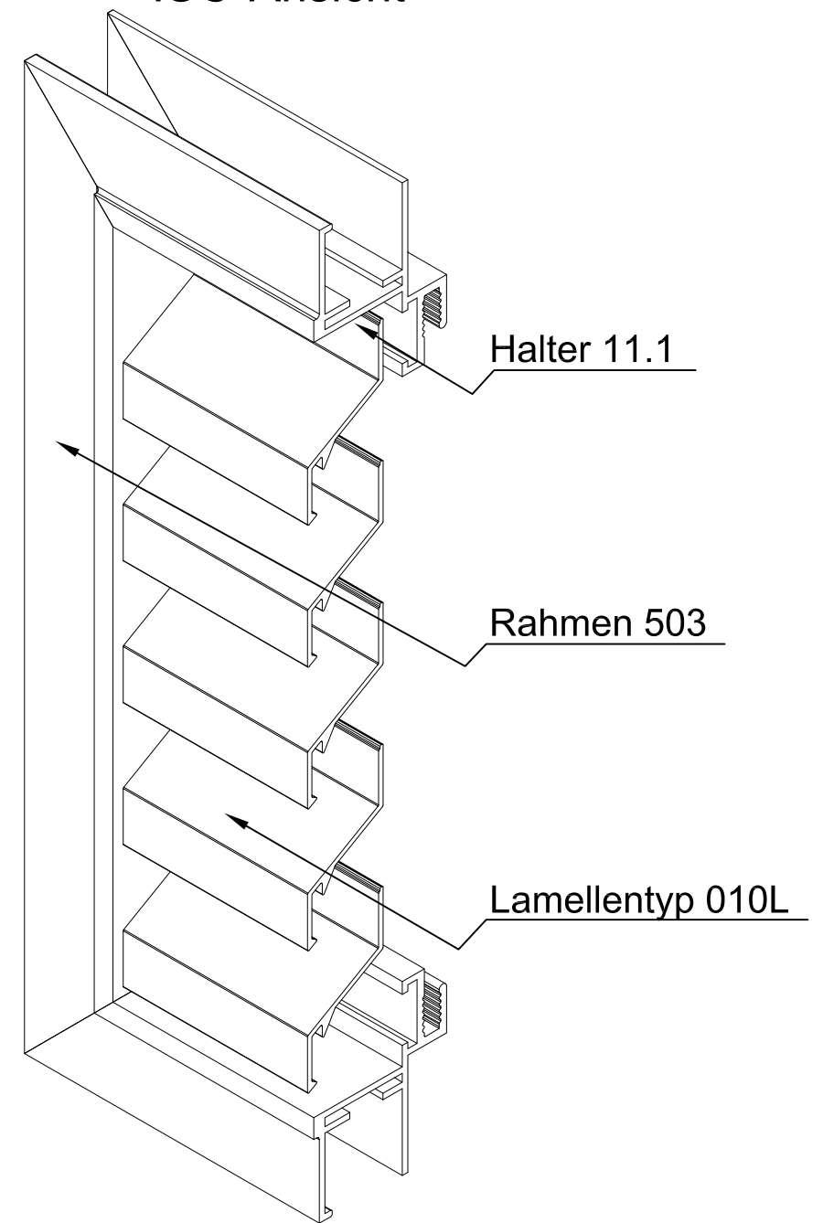
ISO-Ansicht
