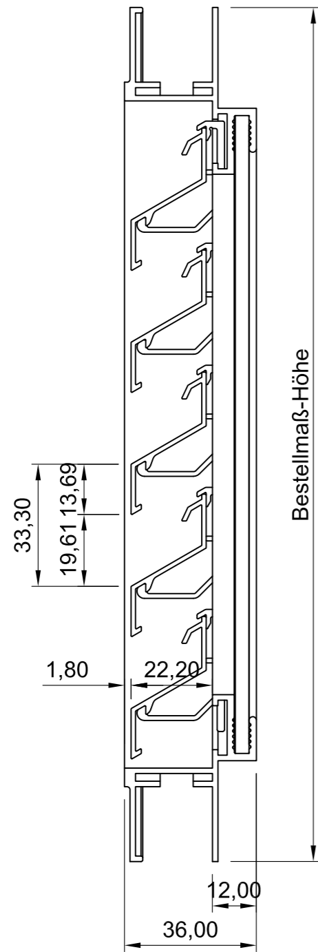
Draufsicht
