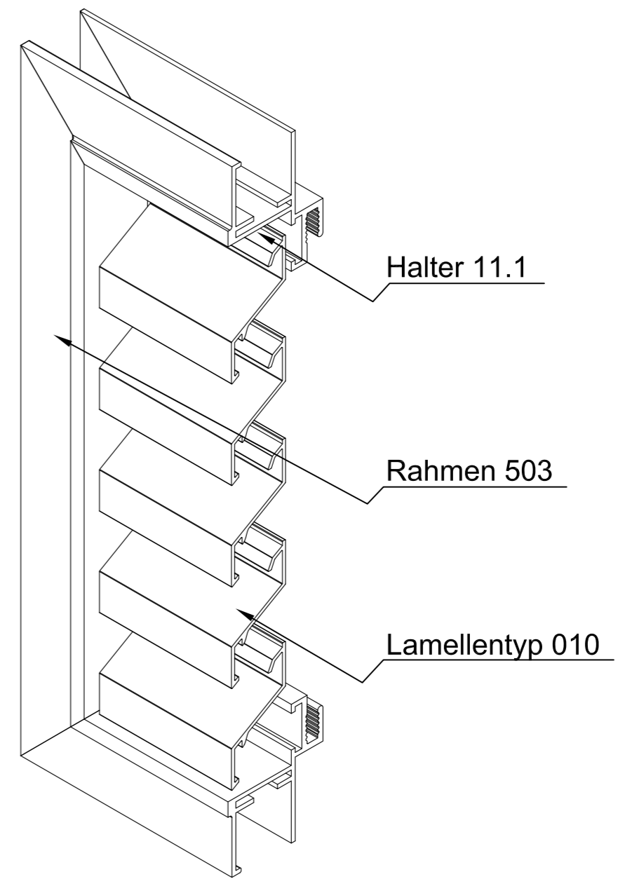
ISO-Ansicht
