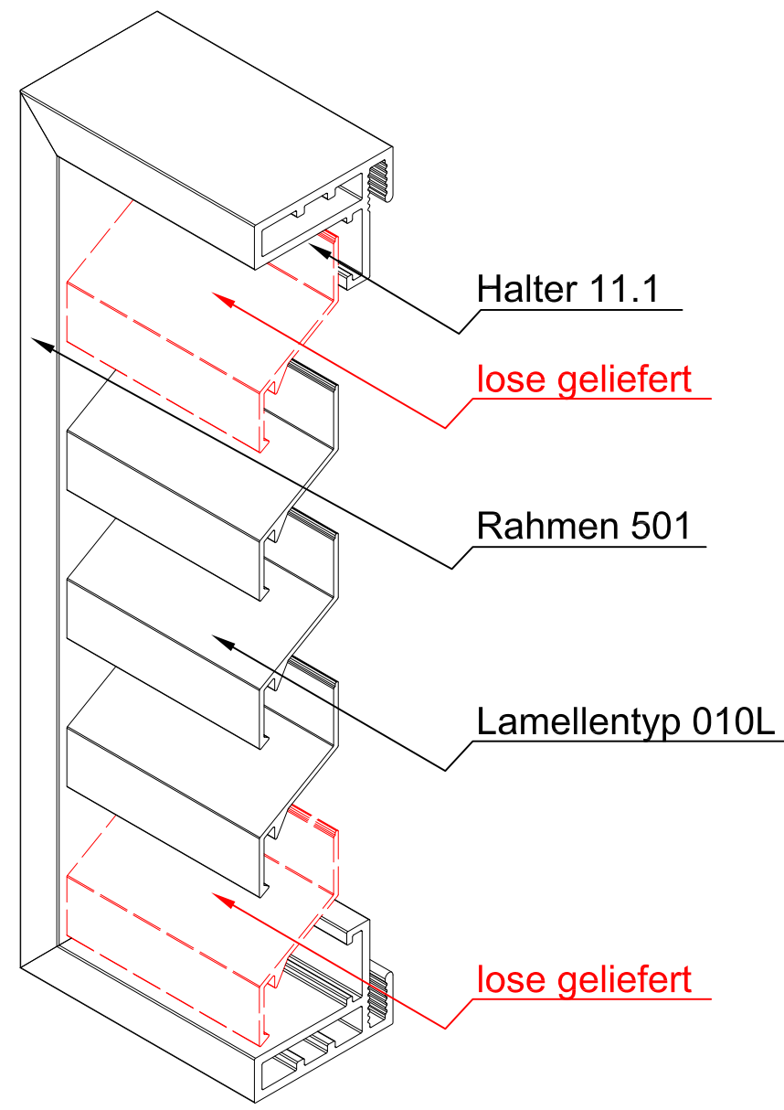
ISO-Ansicht
